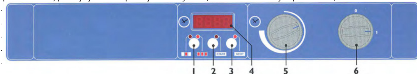
Obr. 1: 1 - hlavní vypínač (jednotky), 2 - indikátor pracování, 3 - tlačítko START, 4 - tlačítko STOP, 5 - regulace teploty, 6 - regulace výkonu
